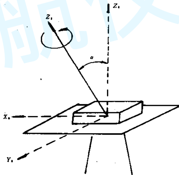
图 2 万向旋转支撑台面
